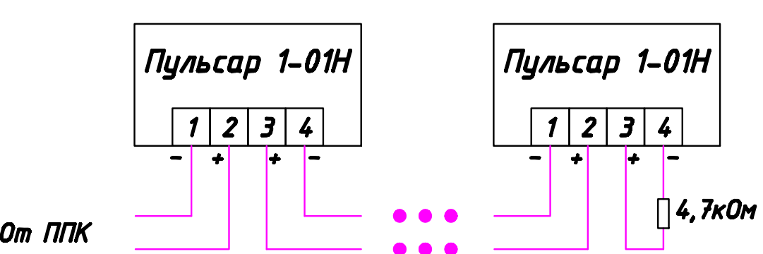
Схема подключения извещателей пламени Пульсар 1-01Н
